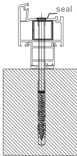
tubular frame anchor
