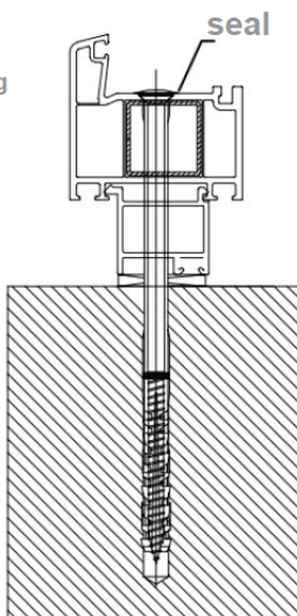
tubular frame anchor
