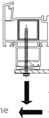
tubular frame anchor
